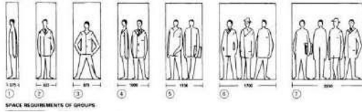
Gambar 8. Standar Kebutuhan Tempat di antara Dinding Sumber : Ernst Neufert (Data Arsitek)
