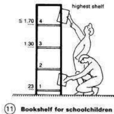
Gambar 7. Standar Rak Buku dan Rak Katalog
