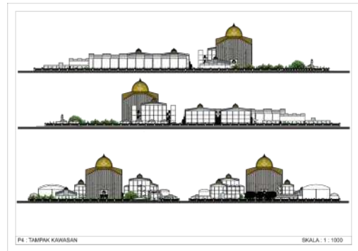
Gambar 27. Gambar tampak kawasan pesantren Sumber : Analisis pribadi
