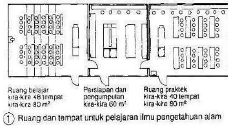
Gambar 10. Standar Ruang Pelajaran Ilmu Pengetahuan Alam Sumber : Ernst Neufert (Data Arsitek)
