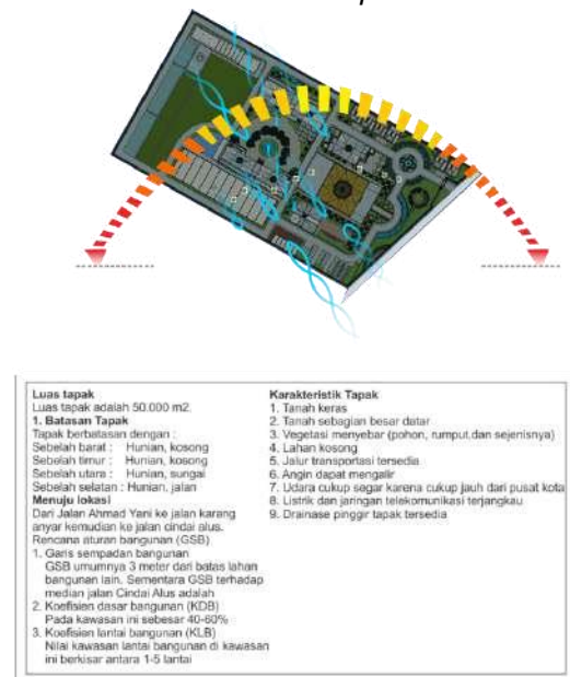
Gambar 13. Lokasi tapak Sumber : Analisis pribadi
