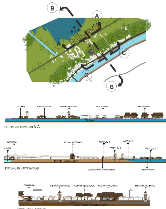
Gambar. 17 Potongan Kawasan Sumber : Analisis Pribadi (2020)
