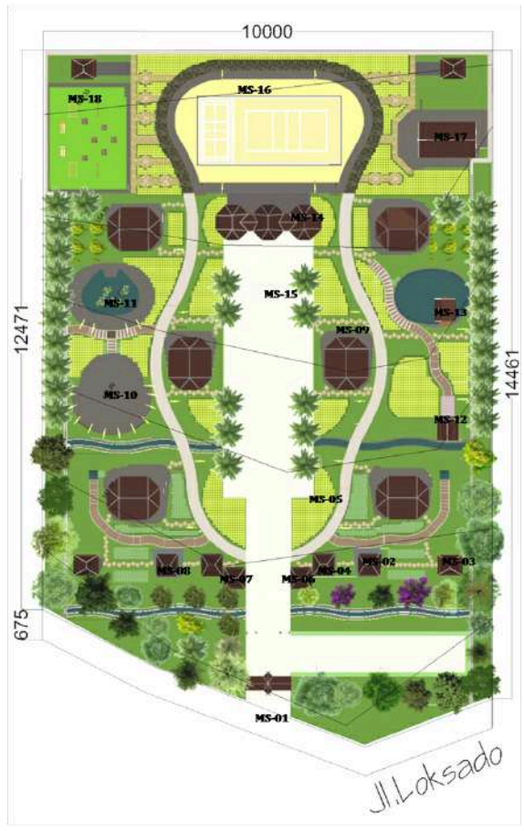
Gambar 3. Rancangan Tapak Sumber : Penulis (2023)
